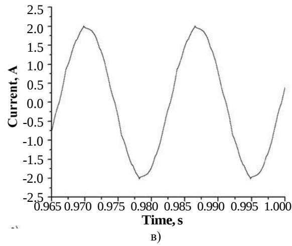
Рис. 6. Зависимости тока от времени: а) — первый слой алгоритма; б) — второй слой алгоритма; в) — третий слой алгоритма
