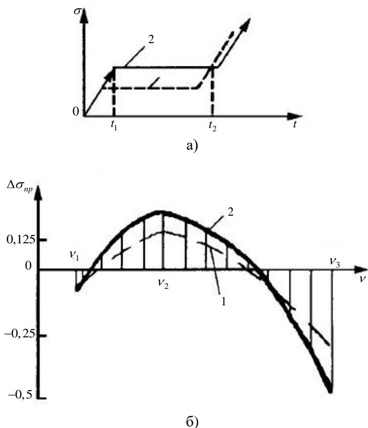
Рис. 6. Результаты теоретического расчета зависимости \sigma_{np}^k / \sigma_{np} от уровня предварительного нагружения для \nu = 2 \cdot 10^7 МПа·с -1 при P = 400 МПа, \lambda = 0,3 (1) и P = 100 МПа, \lambda = 0,3 (2)
