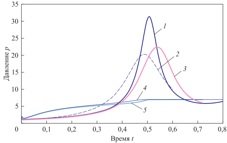
Рис. 6. Давление в кольцевом пространстве при втекании воды p_r (1, 2), p_{втск} (4) без учета деформаций стенок ПК и ЛА и p_r (3), p_{втск} (5) с учетом деформаций; изотермический (—, —, —, —) и адиабатический (---) процессы сжатия газа
