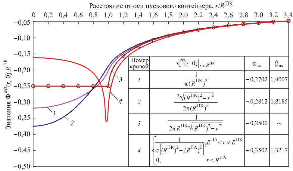
Рис. 4. Поведение единичных потенциалов \Phi^{ext} при z=0 :
